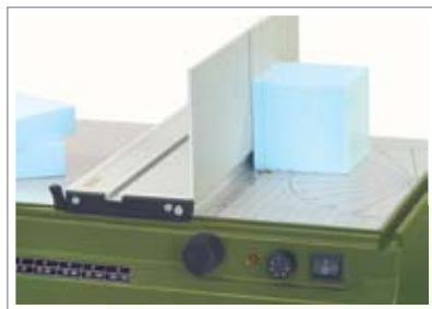
Θερμικός κόφτης THERMOCUT 230/E (Κωδ. 2708000) και οδηγός κοπής TA 300 (Κωδ. XXX) για τη δημιουργία και αναπαραγωγή γεωμετρικών στερεών σε γωνίες 0°-90° και λεπτών φύλλων με απόλυτη ακρίβεια
